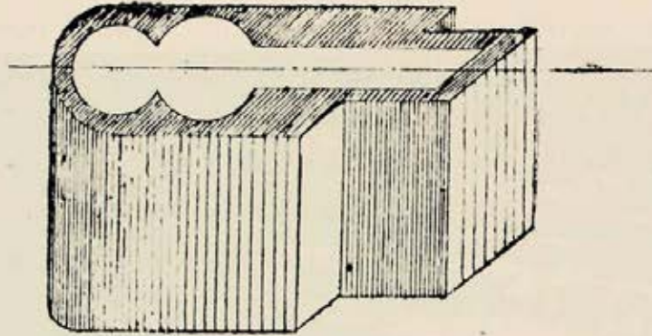
(Εἰκ. 19). Μαρμαρίνη κολυμβήθρα ἐν Βυζαντίῳ παρὰ τὰς Βλαχέρνας (Ἀἰῶν - Σερράϊ), κατὰ σχεδιογράφημα τοῦ κ. Δ. Τρυφίδου.
