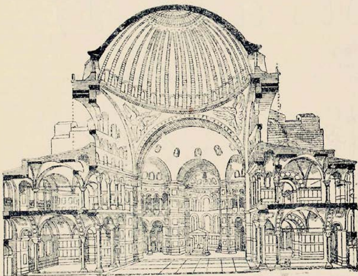
(Εἰκ. 8). Ἐγκάρδιος τομὴ τοῦ Ναοῦ τῆς Ἁγίας Σοφίας κατὰ τὴν ἐκ Βορρᾶ πρὸς Μεσημβρίαν διεύθυνσιν.
